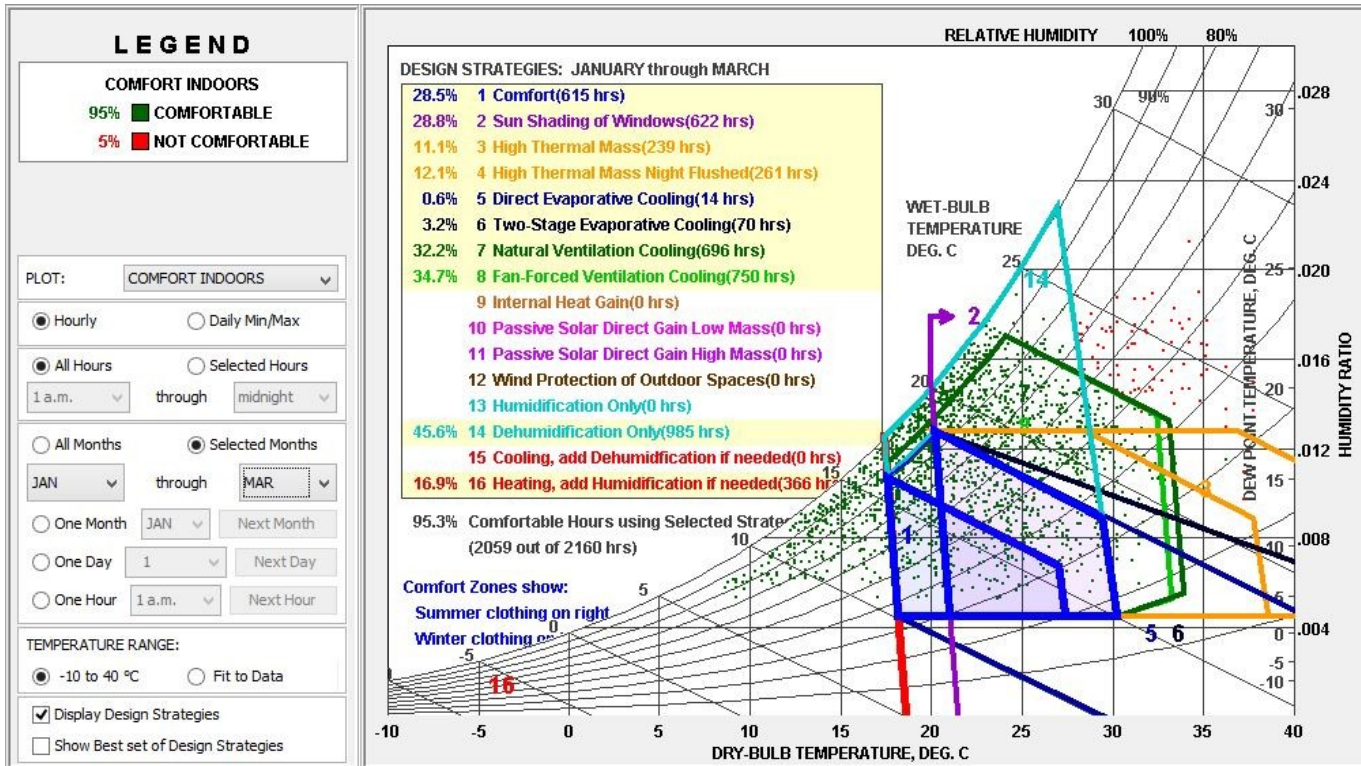
Imagen 25-Diagrama Psicrométrico de los meses de verano
