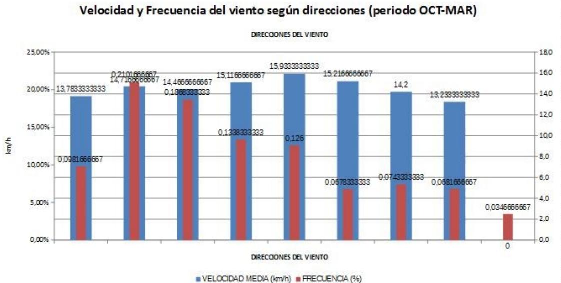
Imagen 14-Velocidad y Frecuencia de vientos VERANO
