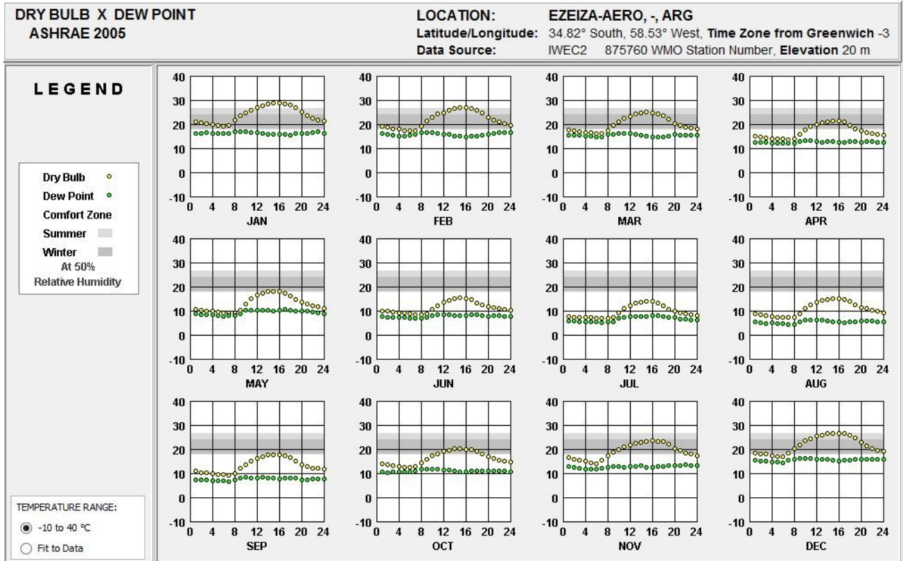
Imagen 24-Diagrama mes a mes de Zonas de Confort
