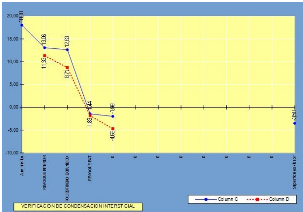
Imagen 37- Gráfico de Condensación de Muro con Bloque H
