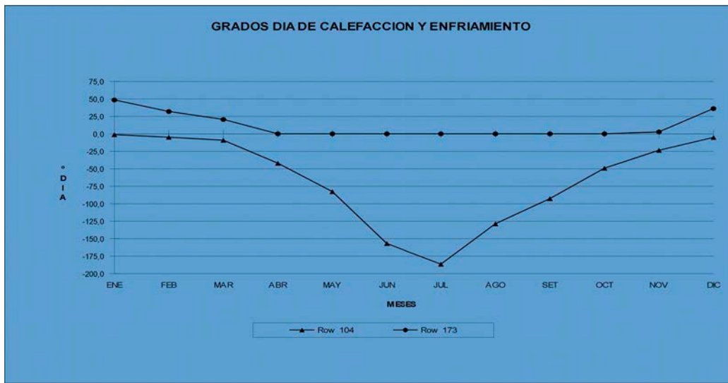
Imagen 11- Grados días de calefacción y refrigeración
