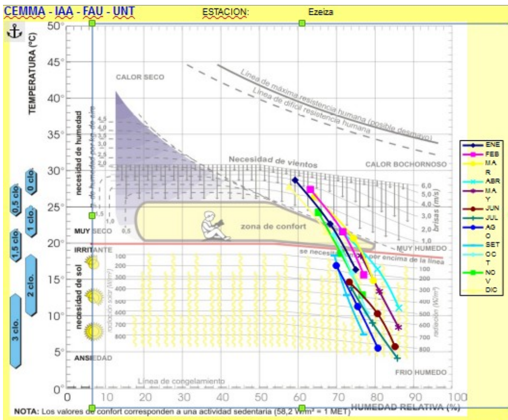
Imagen 19- Diagrama de OLGAY
