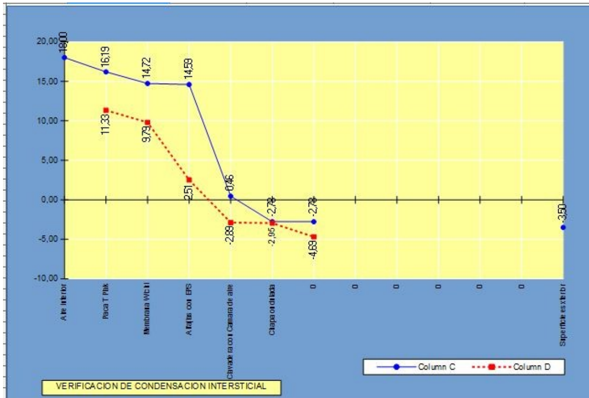
Imagen 38- Gráfico de Condensación de la cubierta existente
