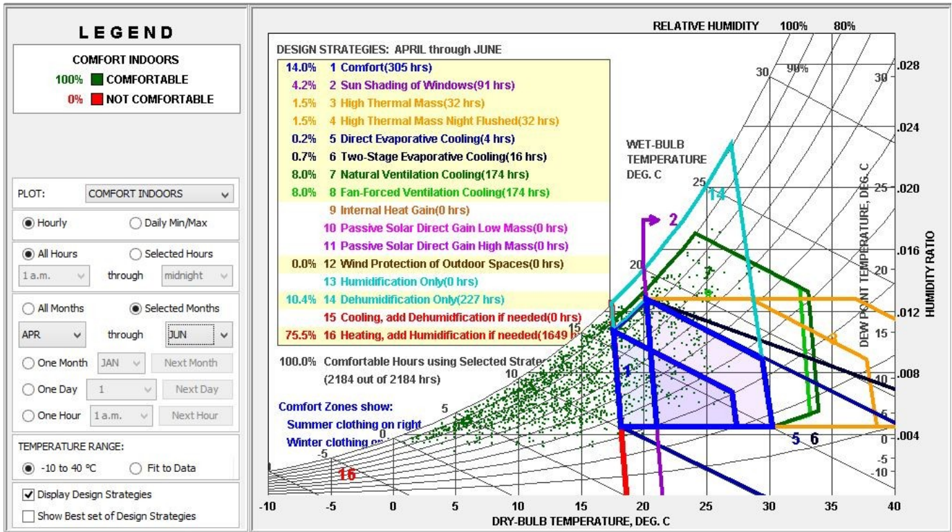
Imagen 26-Diagrama Psicométrico de los meses de otoño
