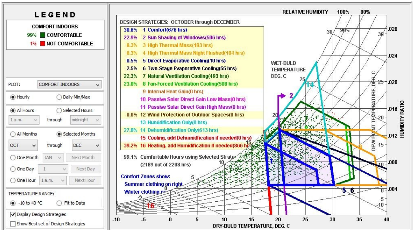
Imagen 28-Diagrama Psicométrico de los meses de primavera
