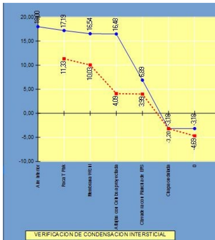
Imagen 41- Gráfico de Condensación de Cubierta Versión Mejorada
