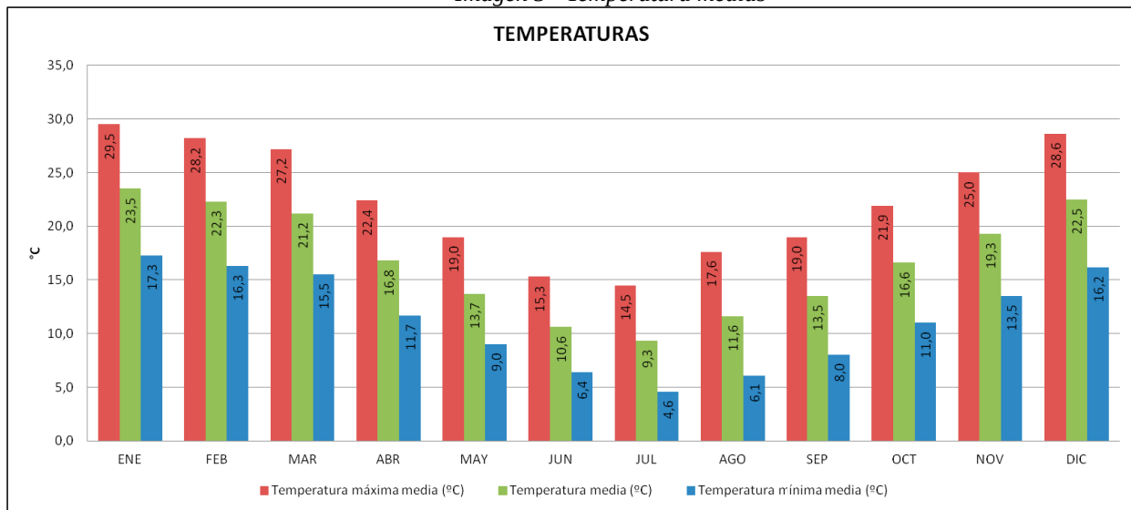
Imagen 6 - Temperatura medias y absolutas
