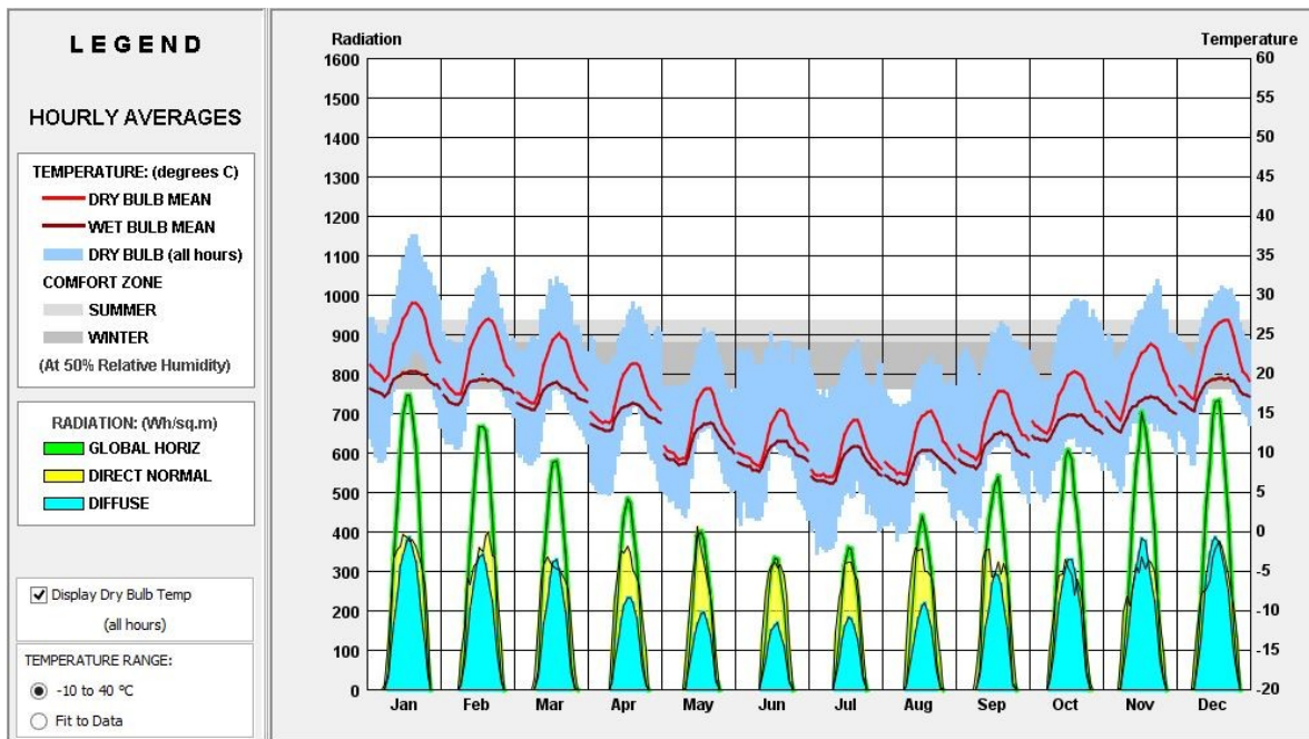
Imagen 22 -Diagrama de Análisis de Radiación y Temperatura mes a mes y zonas de confort
