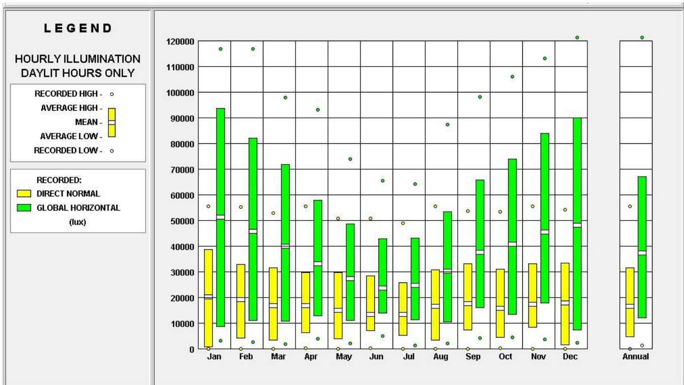
Imagen 23 -Diagrama de Iluminación Natural directa y horizontal en lux
