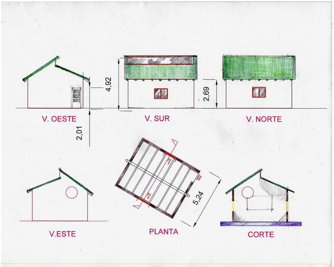
Imagen 29 y 30-Diagrama de Planta General y detalles del Aula
