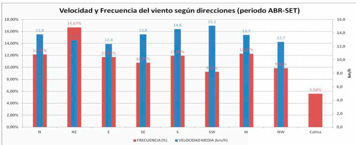
Imagen 15- Velocidad y Frecuencia de vientos INVIERNO
