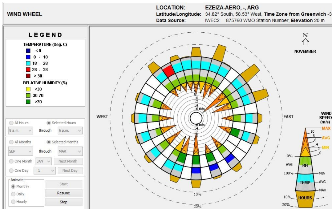
Imagen 56 Análisis de Vientos según Climate Consultant
