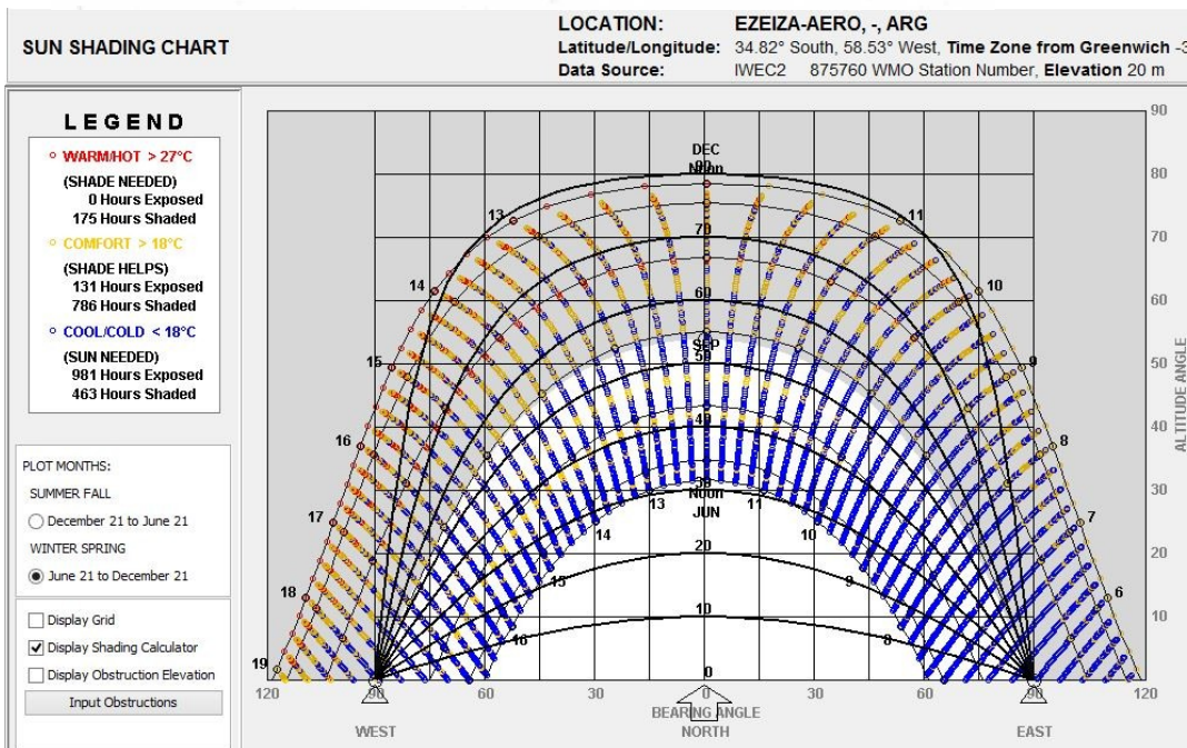
Imagen 48 de Ganancia Solar y Aleros y 49 Aleros según Climate Consultant -
