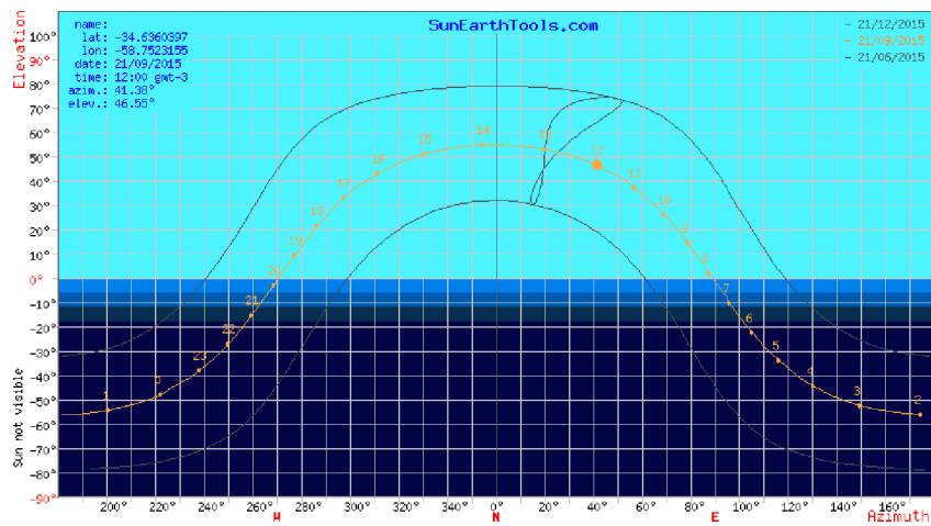
Imágenes 45,46,47 Asoleamiento Invierno, Verano y Primavera
