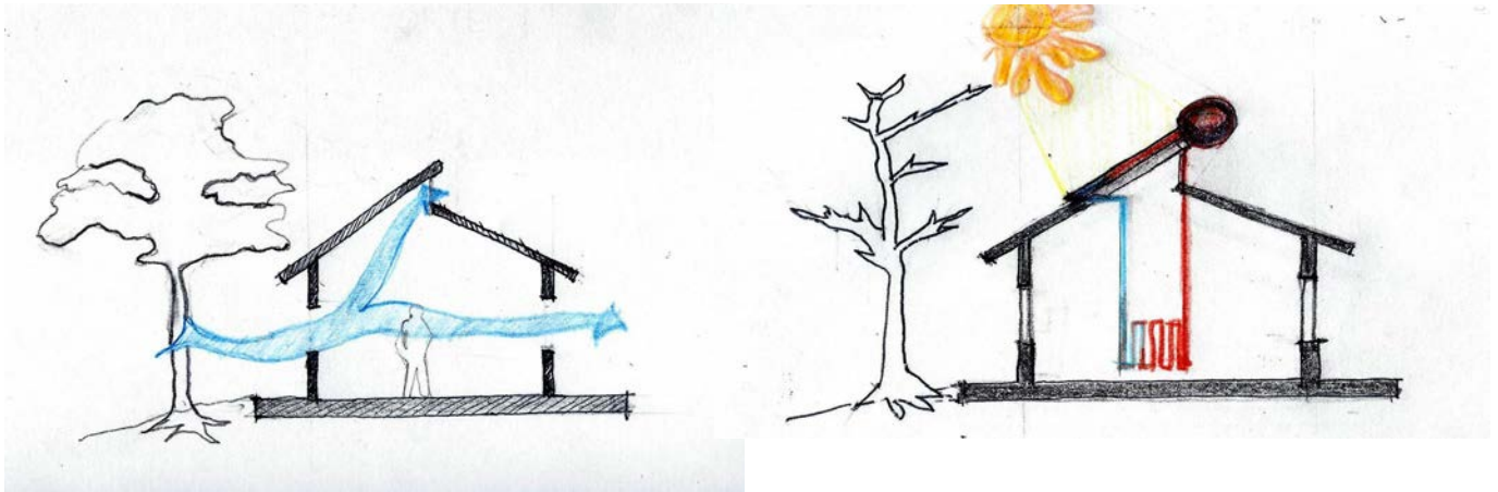
Imagen 54 y 55-esquemas de ventilación cruzada en verano y posible calentamiento solar en invierno
