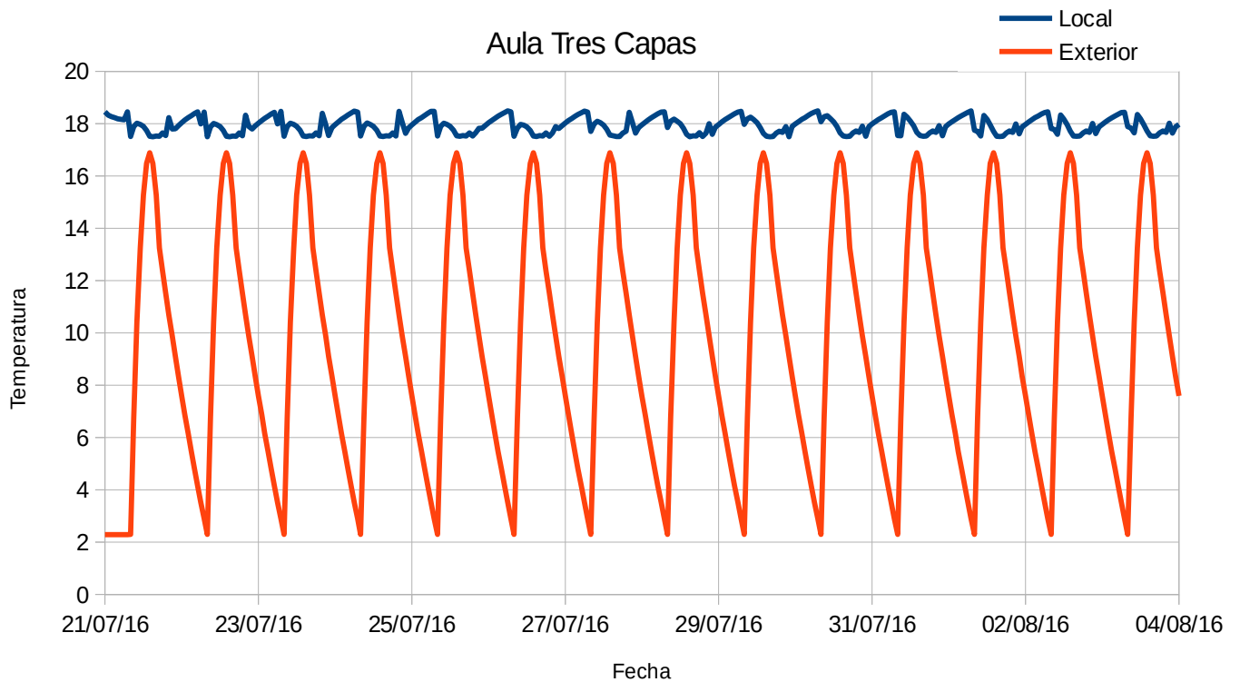
Imagen 42- Gráfico Simedif Versión Mejorada
