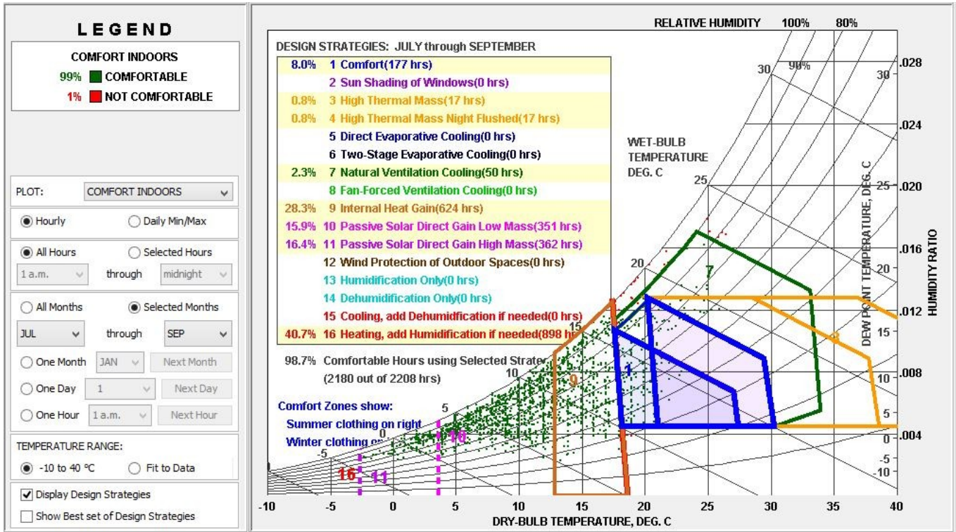
Imagen 27-Diagrama Psicrométrico de los meses de invierno
