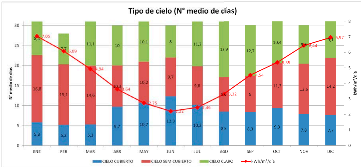
Imagen 16- Radiación y tipo de cielos
